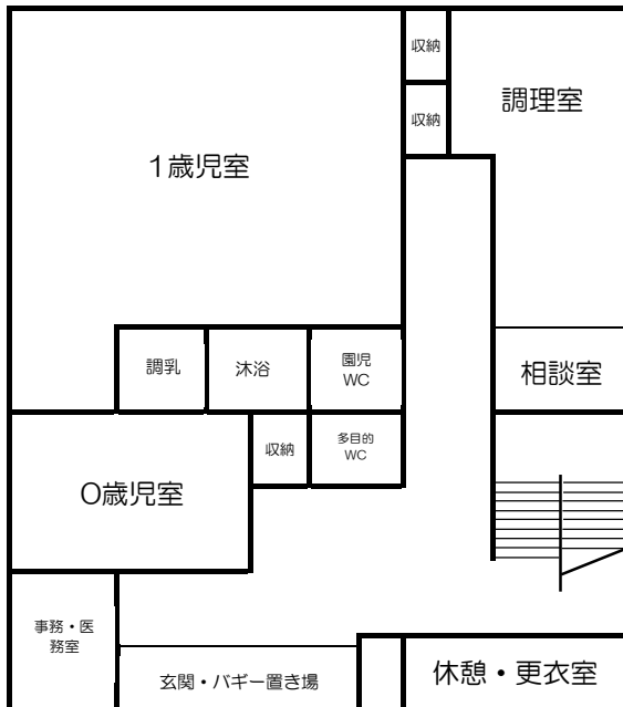
【1階】
